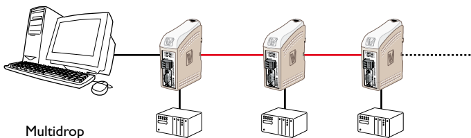
Multidrop
